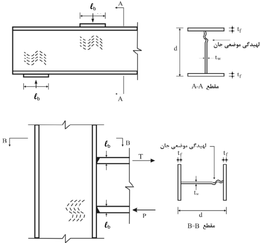
شکل ۱۸-۹-۲-۱۰ لهیدگی جان در مقابل نیروی متمرکز فشاری
