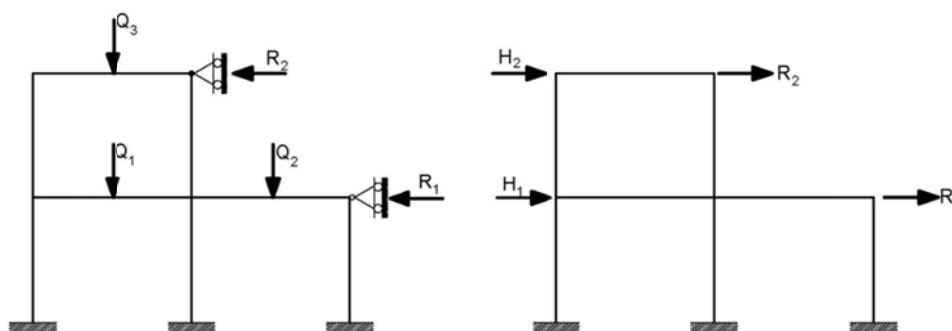
شکل پ-۲-۲ مراحل مختلف تحلیل مرتبه اول قاب برای محاسبه M_{nt} ، P_{nt} و M_{lt} و P_{lt}
